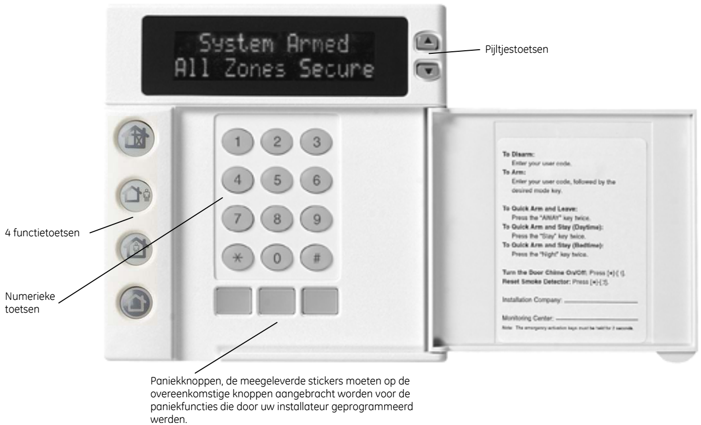
NX-1248 LCD codeklavier
